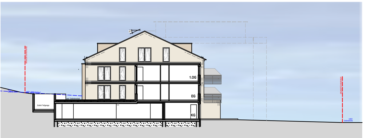
SEITENANSICHT NORD-WEST
